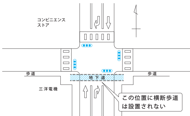
交差点改良工事の概略図（森部地区）
